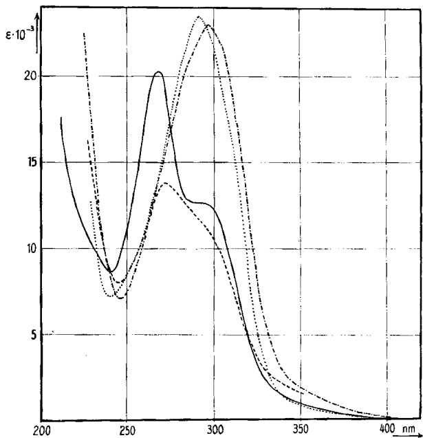
Fig. 4. UV.-Absorptionsspektrum vom Sulfat der Tetrahydrofolsäure (V)
