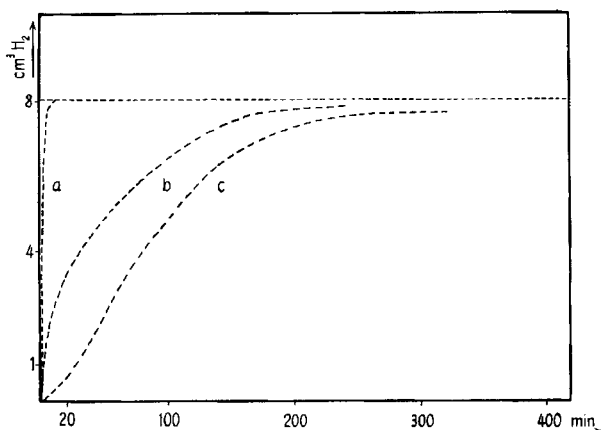
Fig. 3. Hydrierung von Pterin (I) zu 5,6,7,8-Tetrahydropterin (IV) in verschiedenen Lösungsmitteln (Katalysator: \text{PtO}_2 )
