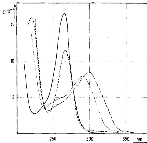
Fig. 2. UV.-Absorptionsspektrum vom Sulfat des 2,4,5-Triamino-6-hydroxy-pyrimidins
