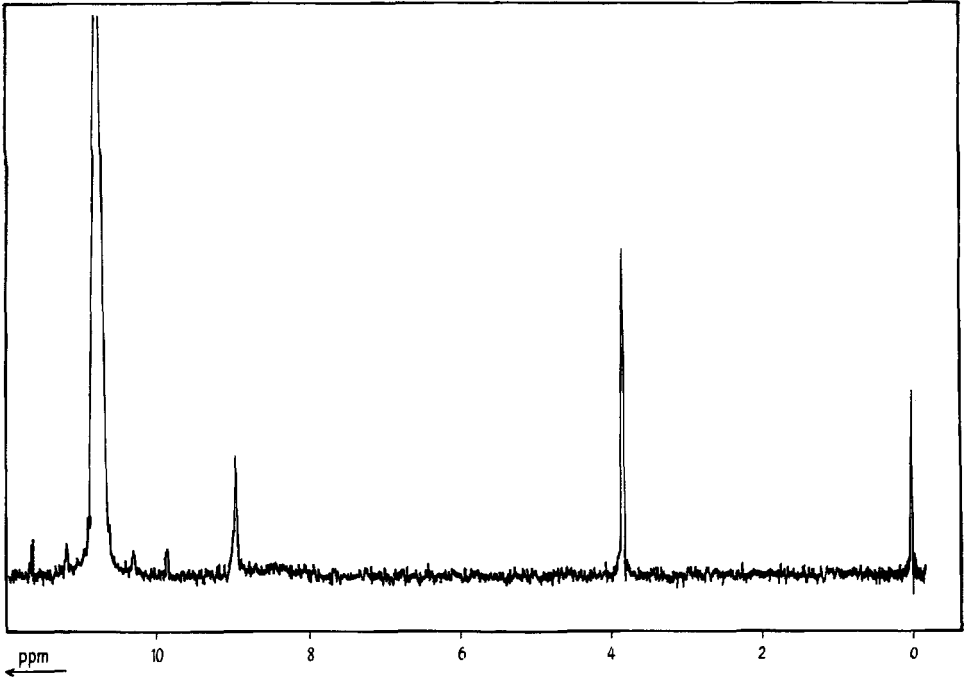
Fig. 5. NMR.-Spektrum von ( N -3)-Methylpterin in CF_3COOH ( \delta_{TMS} = 0 ppm)
