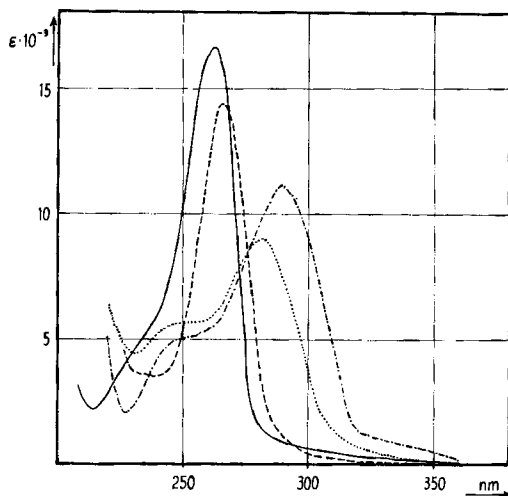
Fig. 1. UV.-Absorptionsspektrum vom Sulfat des Tetrahydropterins (IV)
